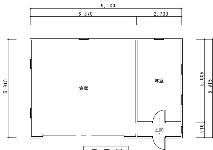
平面図
