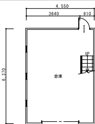
1階 平面図
