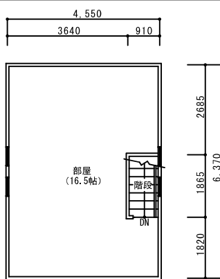
2階 平面図
