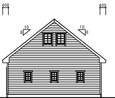
B側立面図
