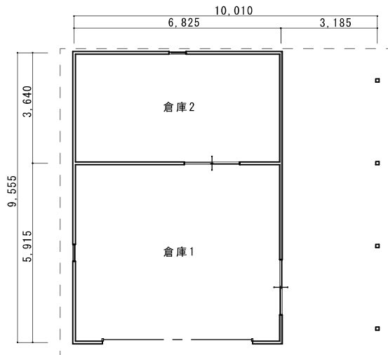
1階平面図
