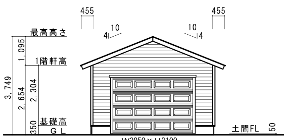
A側立面図
